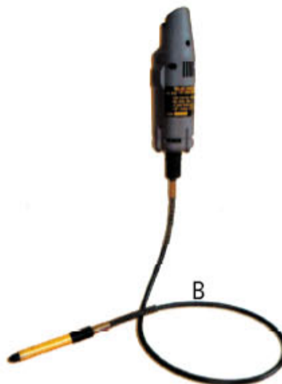
回轉數 : 0~22000PRM 馬力 : 1/5HP(165W) 夾頭能力 : 2.34/3mm
